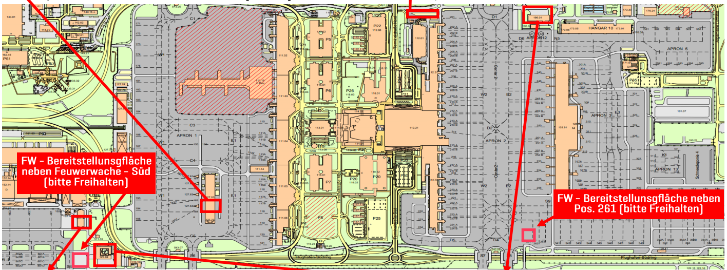
Sperrfläche Feuerwehrzufahrt [RGS2]
